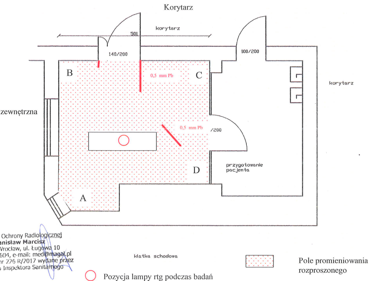
Rys. 2. Osłony stałe i ruchome przed promieniowaniem X dla sali endoskopowej Kliniki Hematologii, Nowotworów Krwi i Transplantacji Szpiku USK we Wrocławiu, ul. Wybrzeże Pasteura 4
